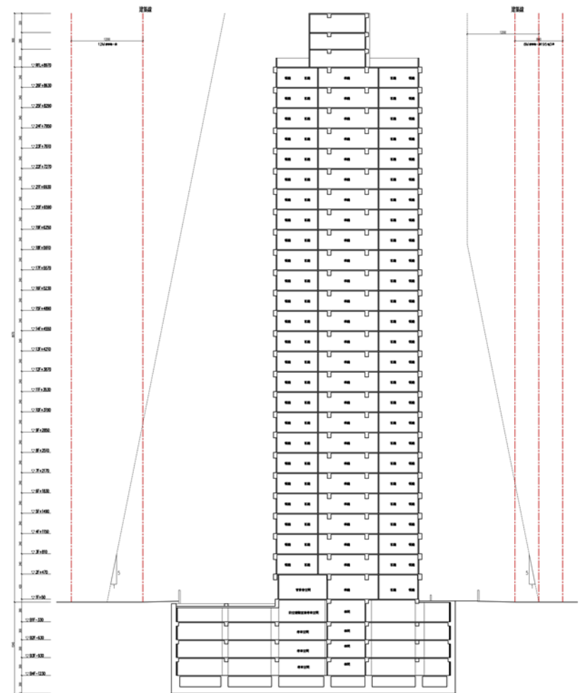
縱向剖面圖
